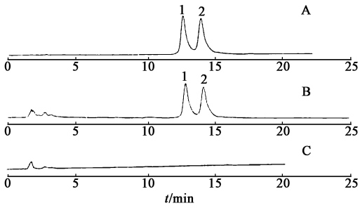
A. 对照品;B. 样品;C. 阴性;1. 补骨脂素;2. 异补骨脂素 图 1 专属性考察 HPLC
