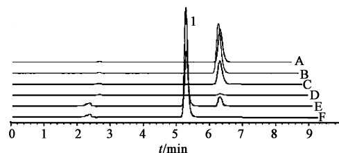
A. 5% 氮酮样品;B. 5% 丁香油样品;C. 空白基质; D. 鼠皮透过液;E. 样品透过液;F. 对照品;1. 磷酸川芎嗪
