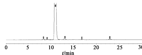
图 9 供试品色谱
