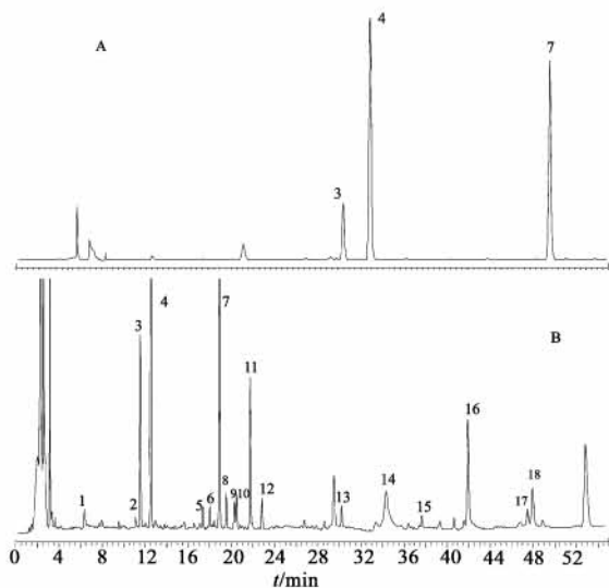
图 1 三七配方颗粒 HPLC
