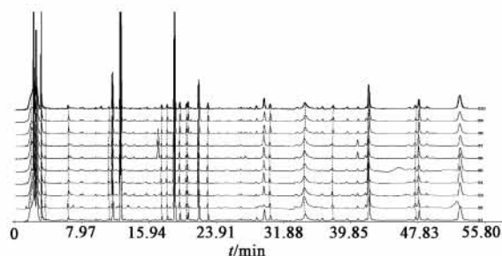
图 2 10 批样品匹配色谱
