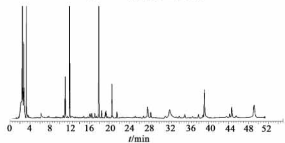
图 3 对照品指纹图谱
