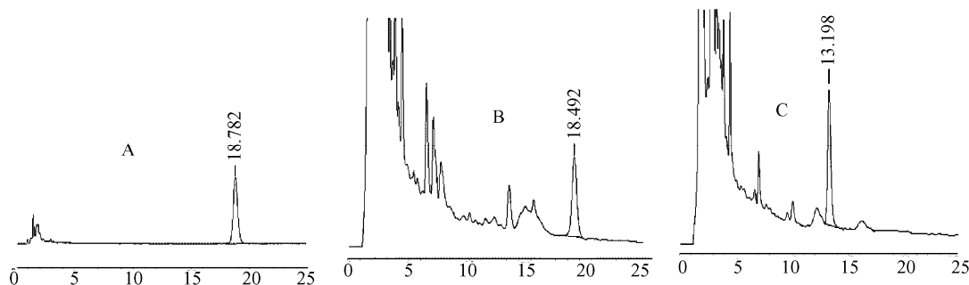
图 1 中耳炎颗粒中连翘苷的 HPLC 图谱
